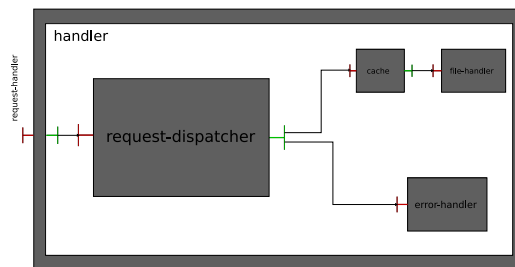
Figure 2. Introduction d'un cache de fichiers dans Comanche.
